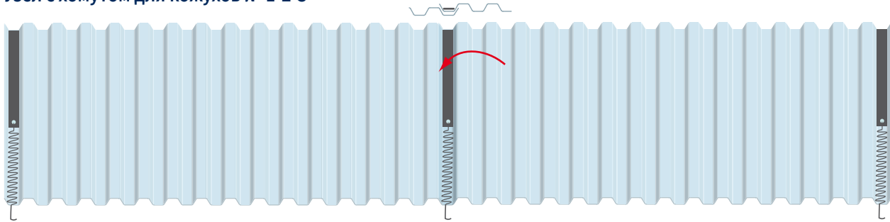
Узел с хомутом для кожуха № 4
